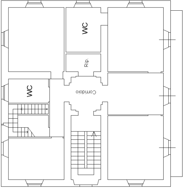
PIANO PRIMO H=4.00
