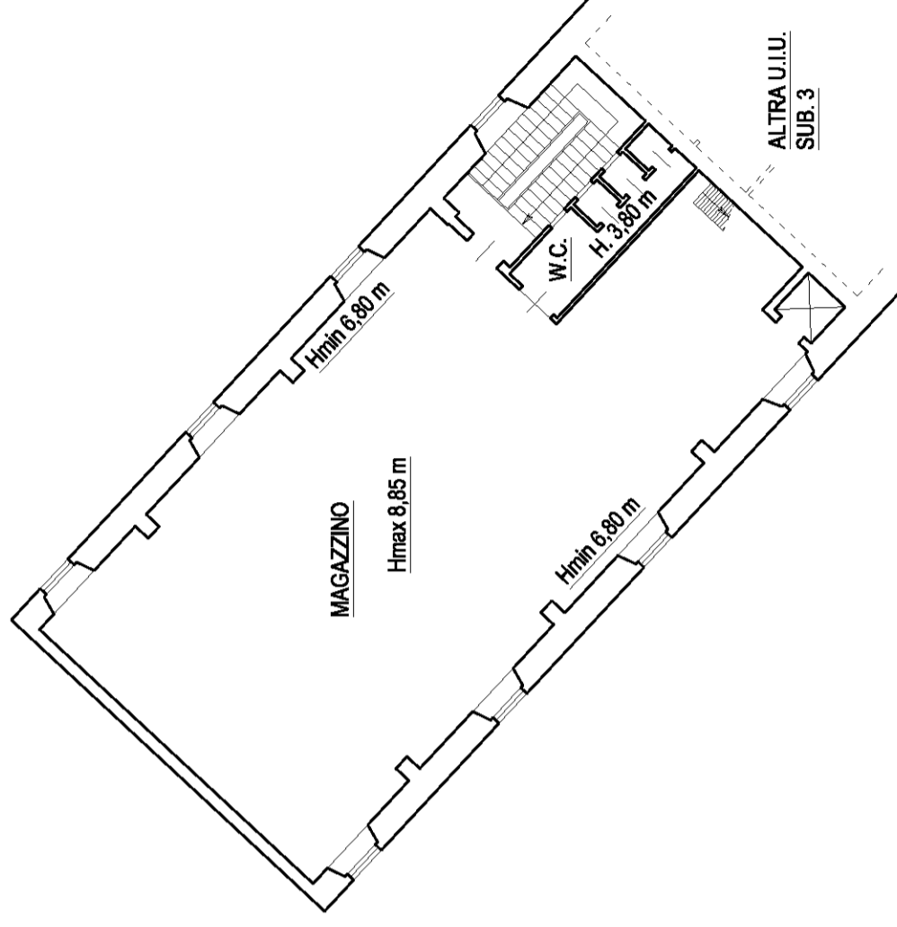
PIANTA PIANO SECONDO Hm. 7,80 m
