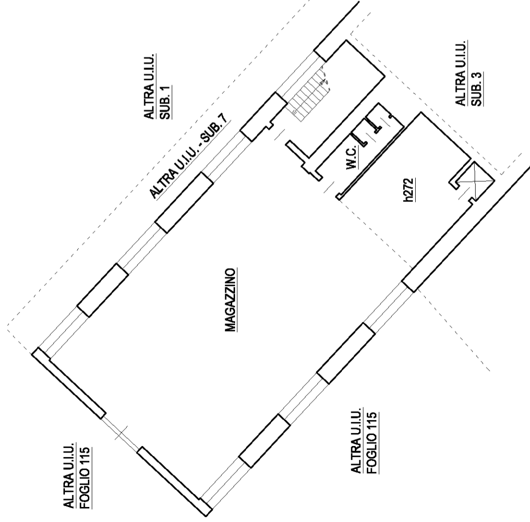
PIANTA PIANO TERRENO H. 7,95 m
