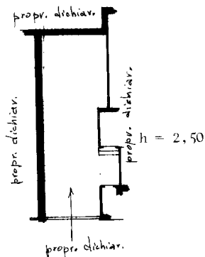
PIANO 1° SOTTOTERRA
