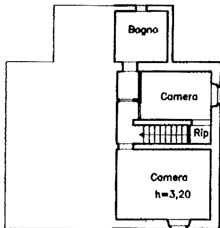
Piano Primo
