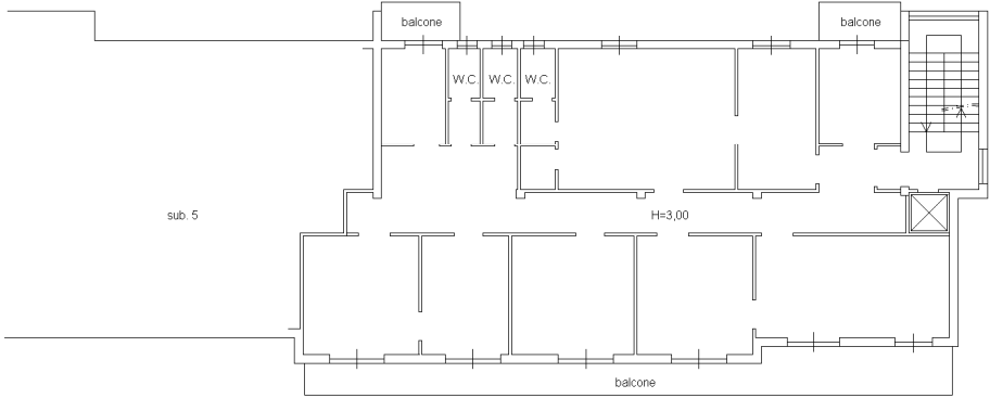
PIANO TERZO
