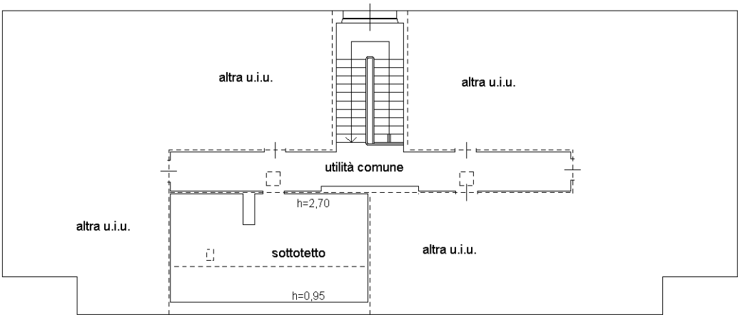
Piano sottotetto hm 1.82m
