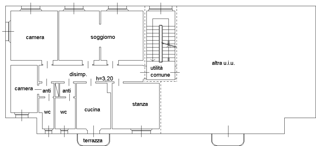
Piano primo h 3.20m
