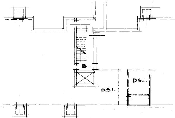
PIANO INTERRATO H. 2.50
